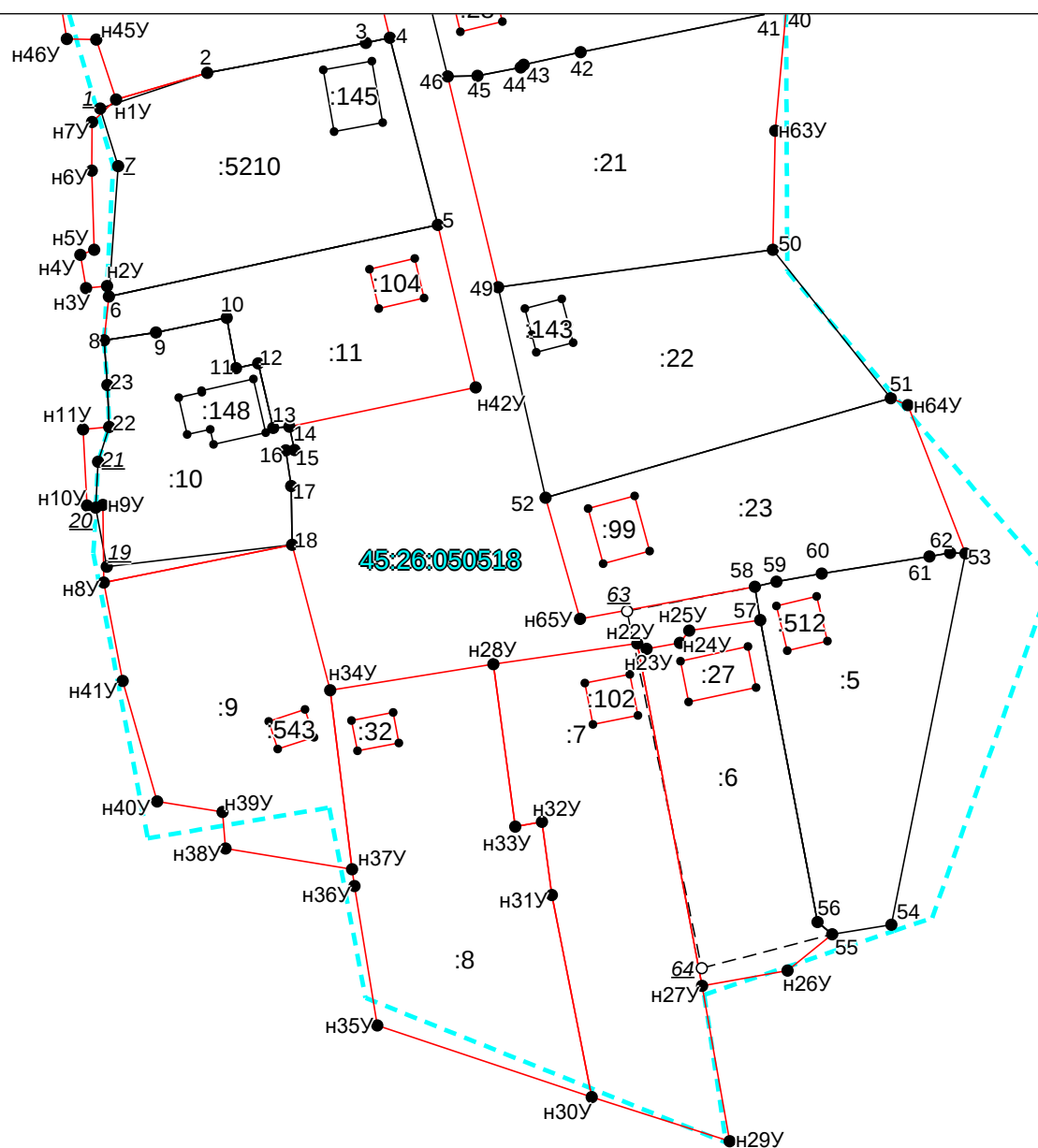
Выносной лист №2
